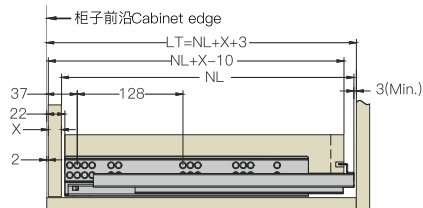
内置抽屉 Internal drawer
